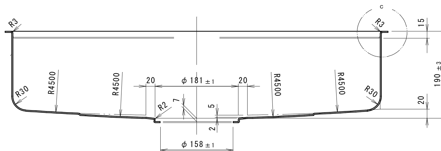
A-A 断面図
