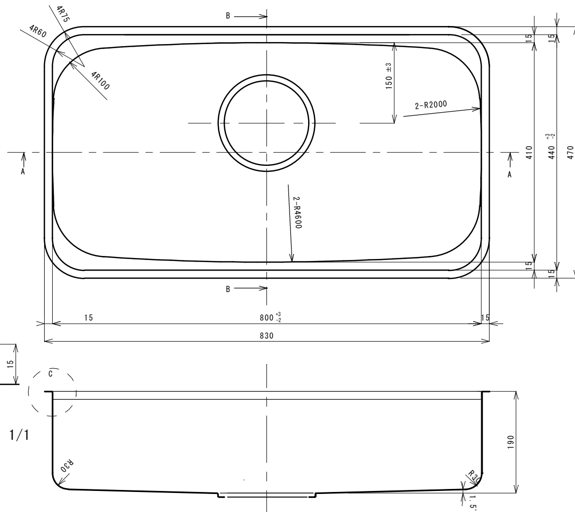
A-A断面図
